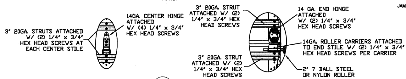
INSIDE ELEVATION N.T.S.
